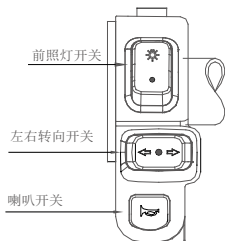
左组合开关
